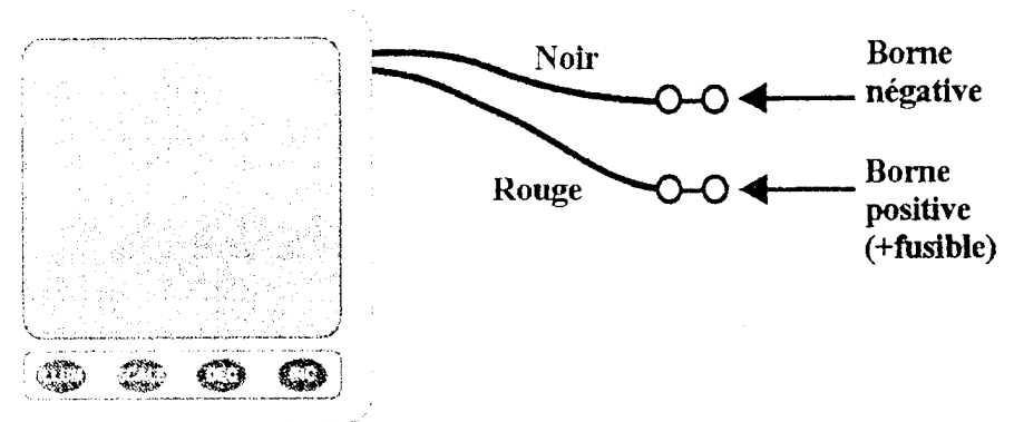
Figure 1 : Alimentation de l'afficheur
